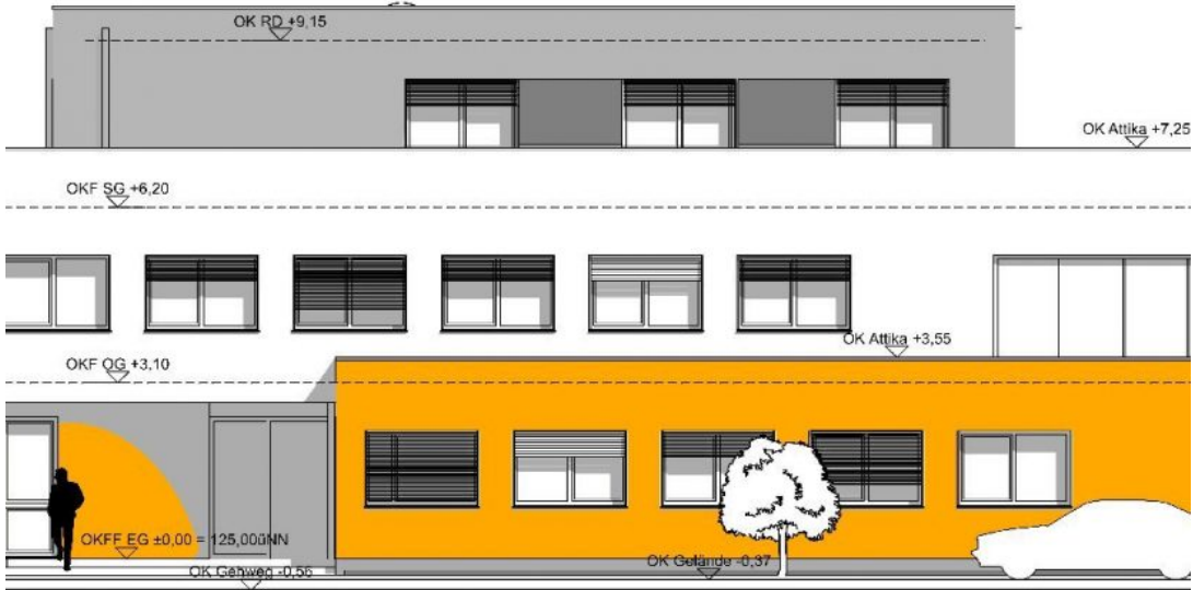
N-WESTANSICHT (STRASSE)
