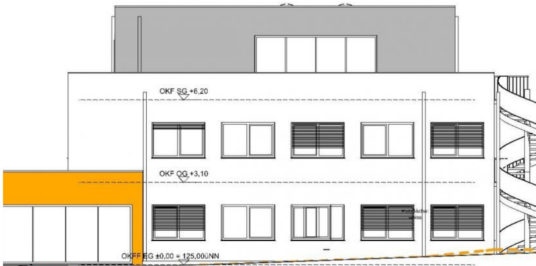
ÜD-OSTANSICHT
