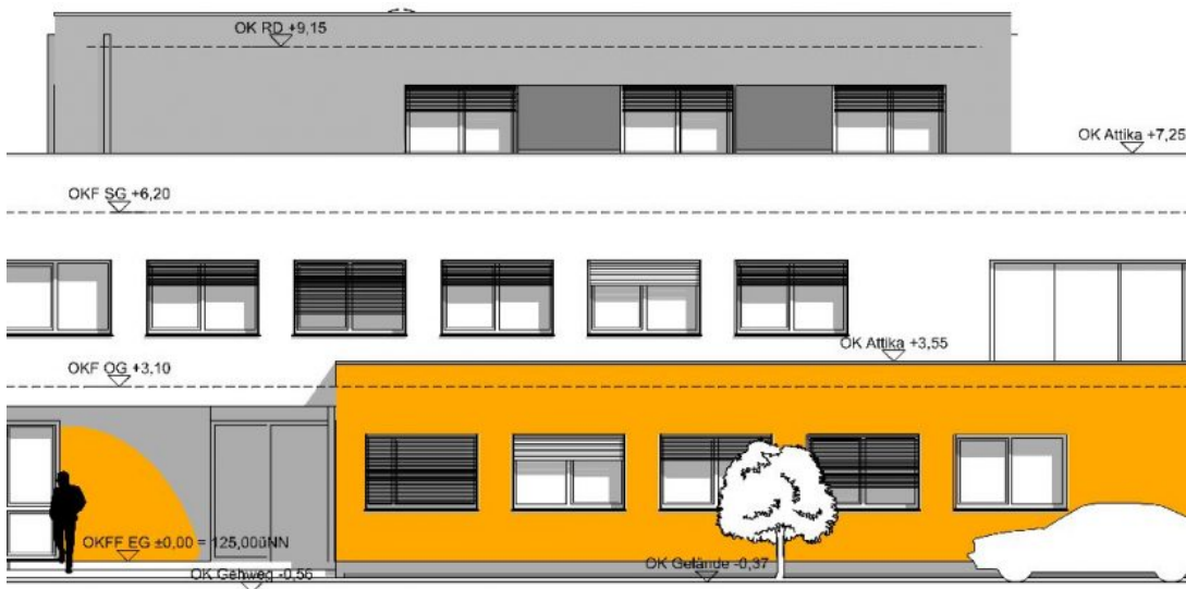
SÜD-WESTANSICHT (STRASSE)
