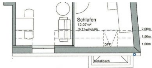
DG Wohneinheit 4.1 2 - Zimmer Wohnung mit Freisitz Wohnen Essen Kochen, Schlafen, AR, Bad mit Dusche, Diele
